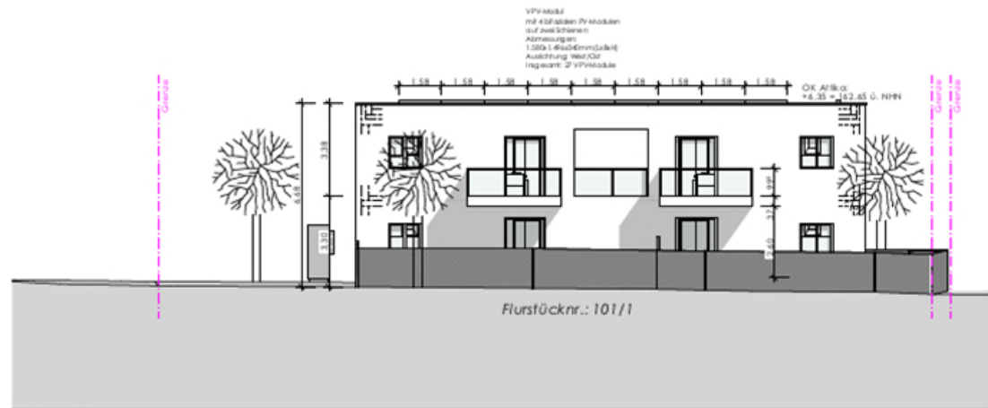
ANSICHT WEST
