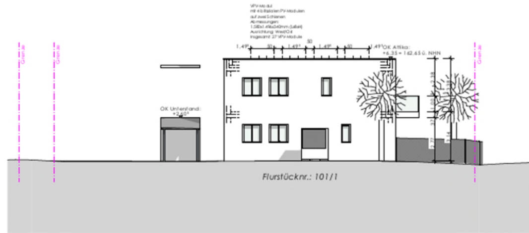
ANSICHT NORD
